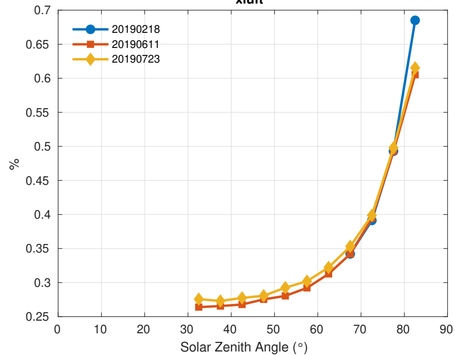
xluft
