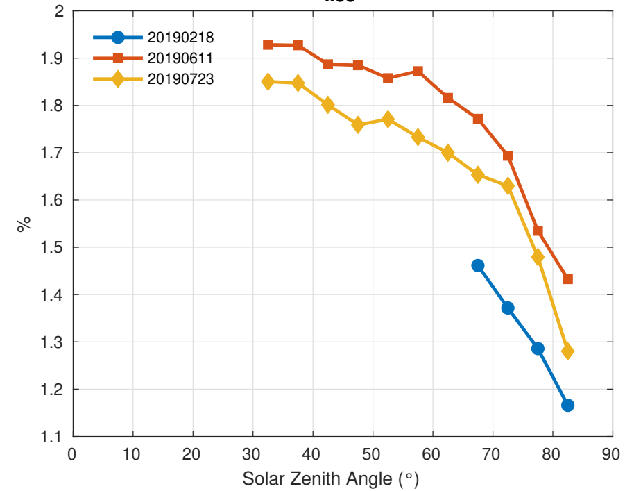
xco
