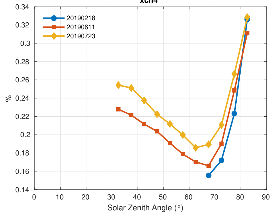
xch4
