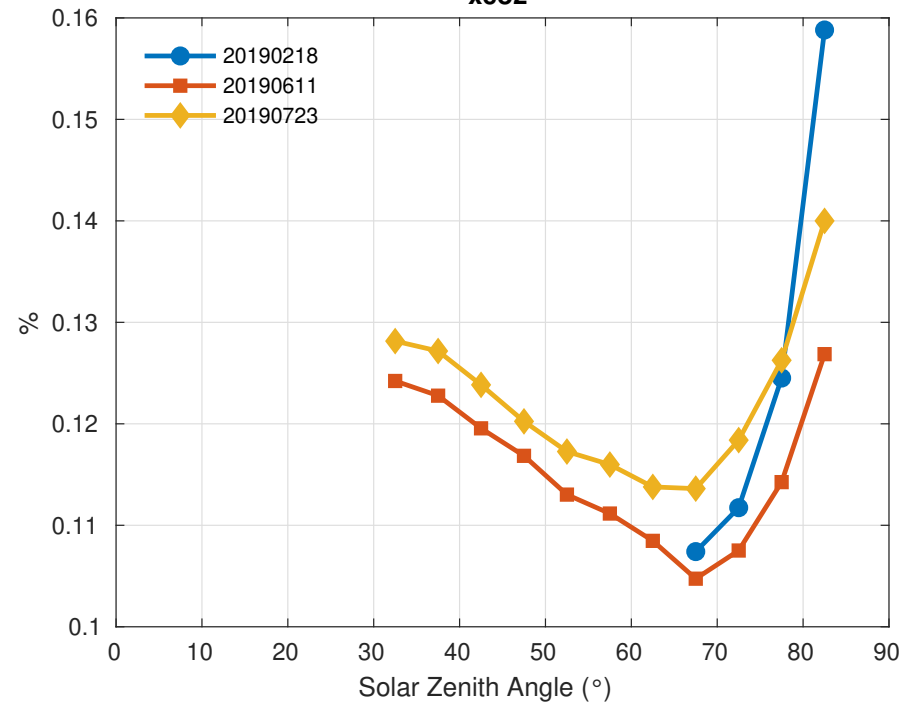
xco2
