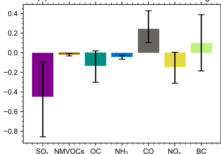
(d) SLCF contributions to 1750-2018 warming
